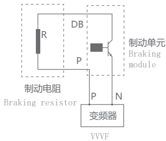
典型电路图
